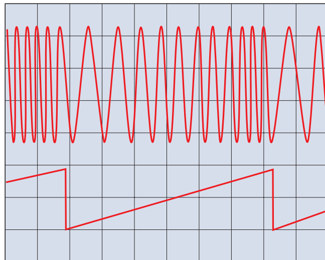
Bild 7: Gewobbelter Sinus; Sägezahnangang
